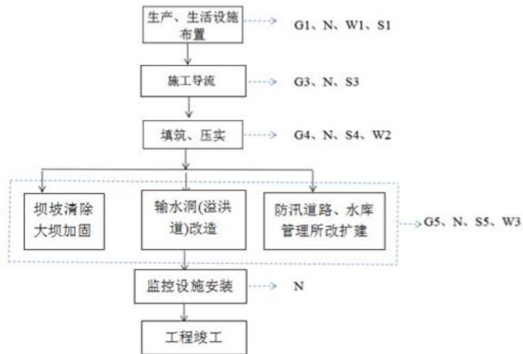
图 4-2 施工工艺流程图
